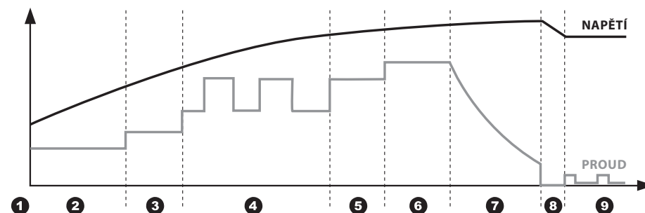
Obr.8, nabíjecí profil nabíječek Extol® Premium 8897300 a 8897301
